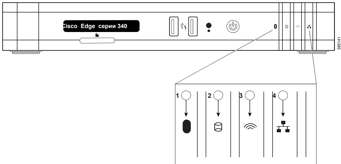
Рис. 5 Светодиодные индикаторы на передней панели устройства Cisco Edge серии 340
