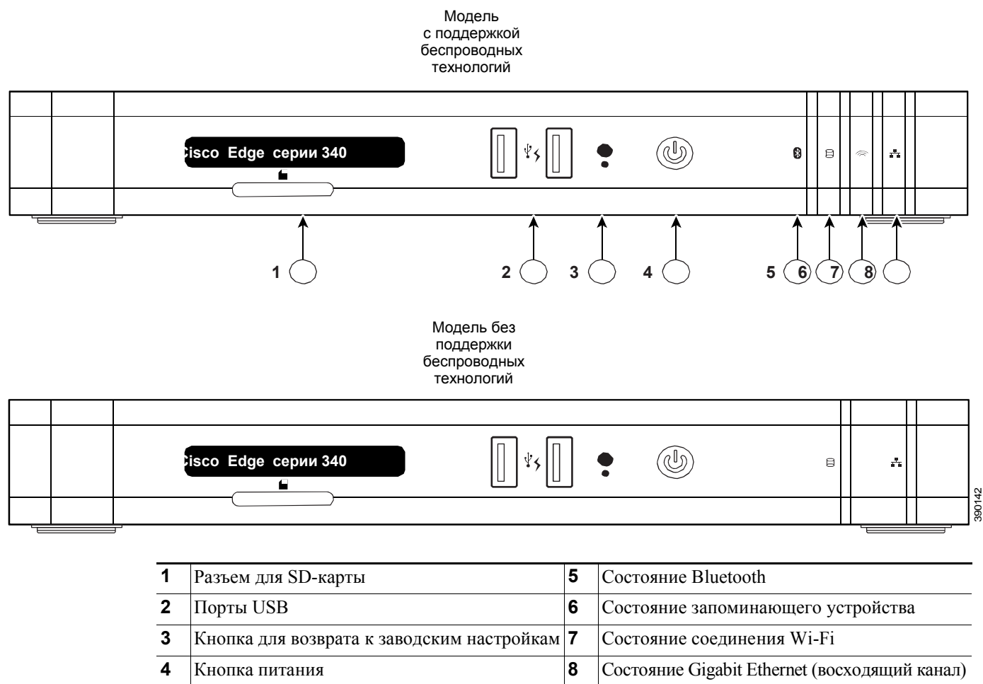
Рис. 1 Cisco Edge серии 340 — Передняя панель
