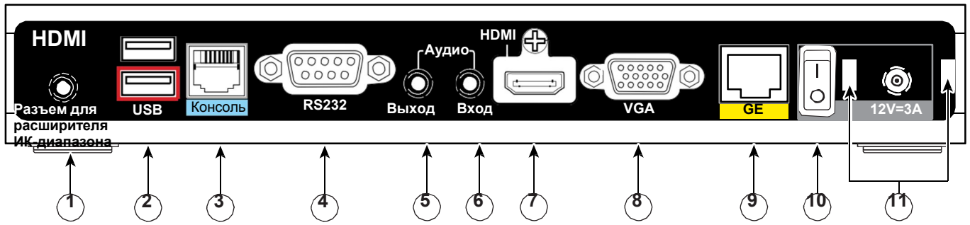
Рис. 2 Cisco Edge серии 340 — Задняя панель
