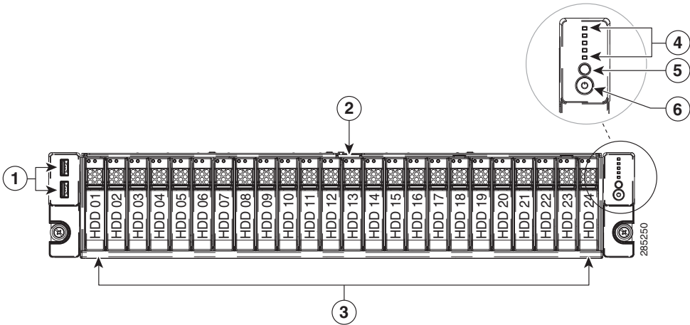
Рисунок 1 Элементы передней панели сервера Cisco UCS C24 M3 (диски SFF)
