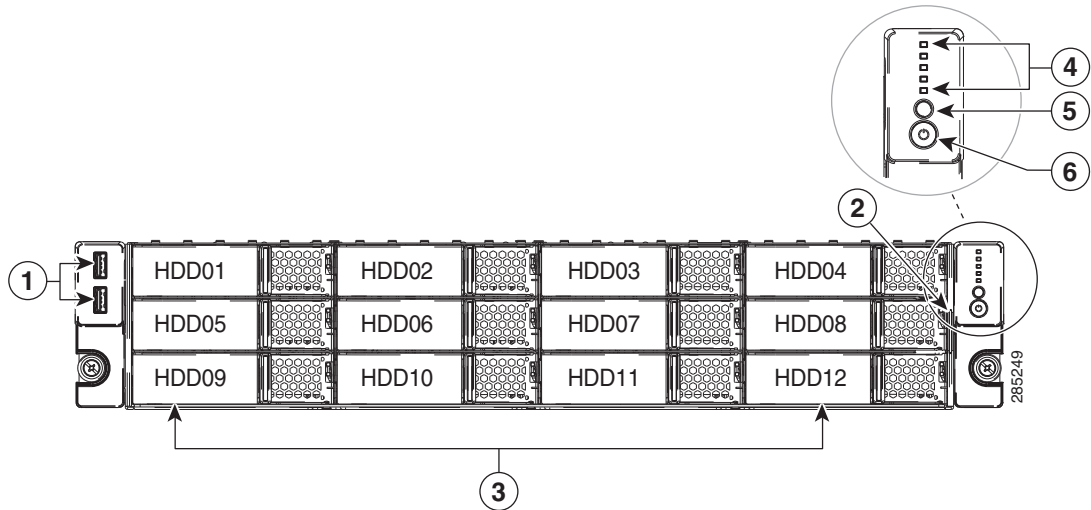
Рисунок 2 Элементы передней панели сервера Cisco UCS C24 M3 (диски LFF)
