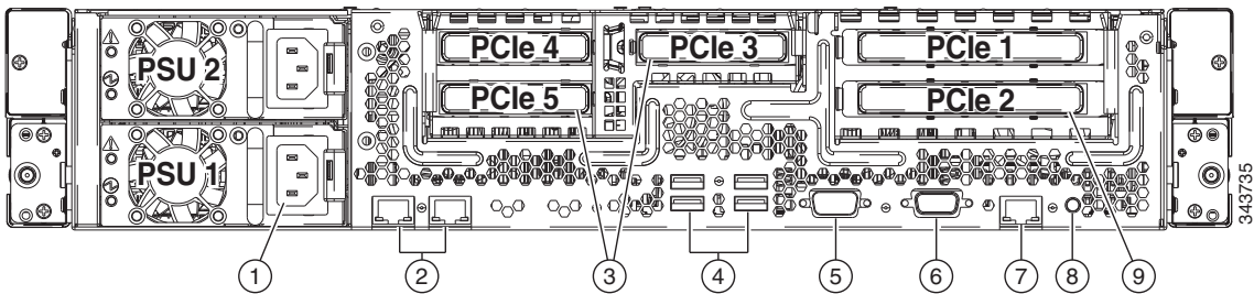
Рисунок 3 Элементы задней панели сервера Cisco UCS C24 M3
