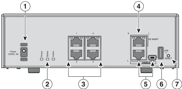
Рисунок 1-1 Задняя панель ASA 5506H-X
